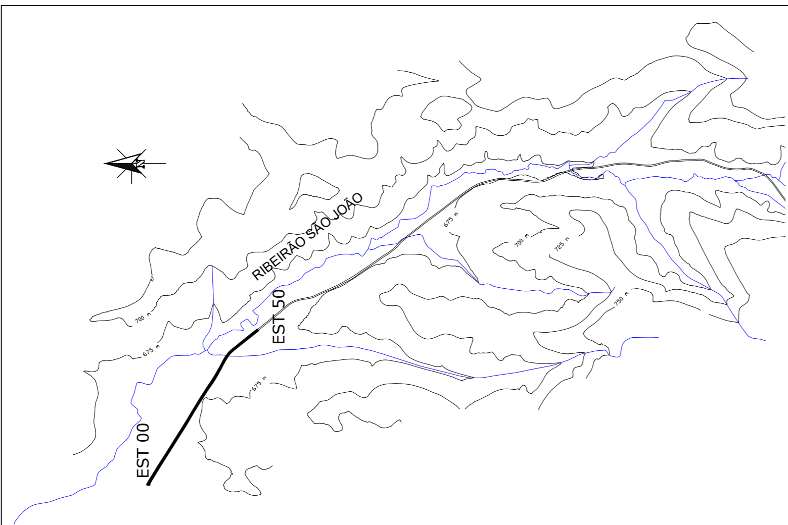
LEVANTAMENTO PLANIALTIMÉTRICO ESC 1:20.000
