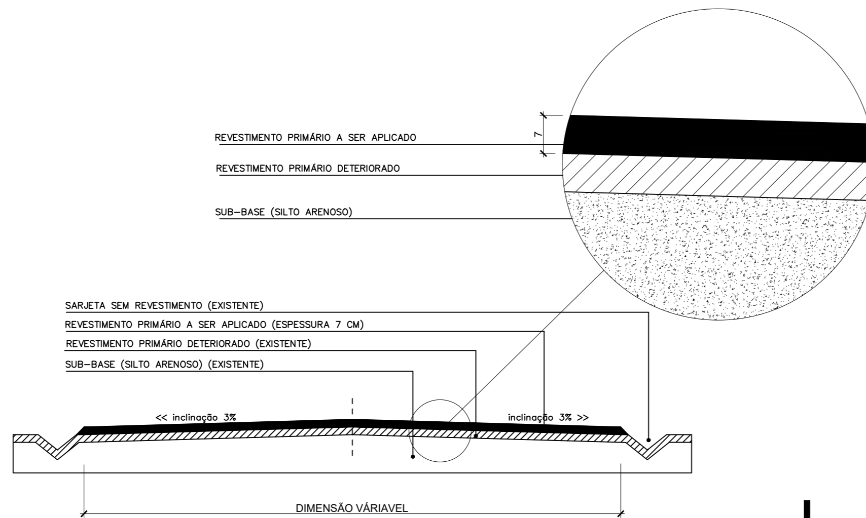
SEÇÃO TRANSVERAL SEM ESCALA
