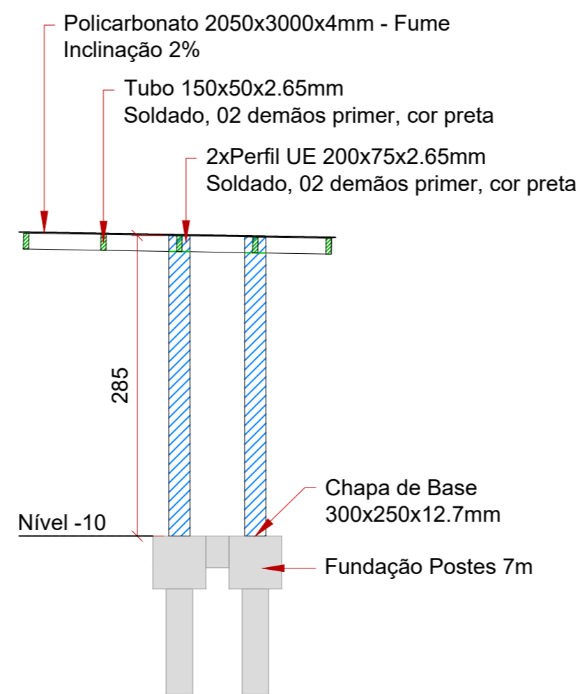
CORTE ESC.: 1:50
