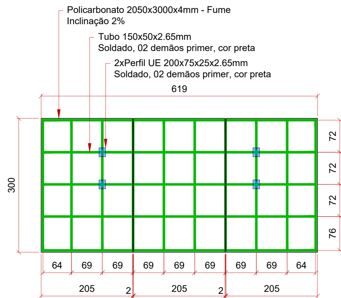
PLANTA ESC.: 1:50
