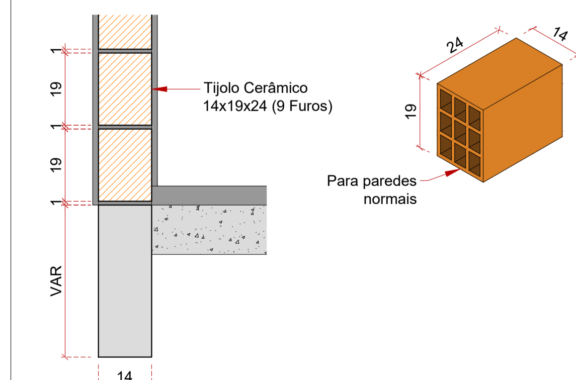
ALVENARIA DE VEDAÇÃO ESC.: 1:10
