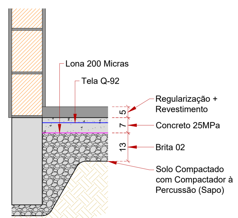
CONTRAPISO ESC.: 1:10
