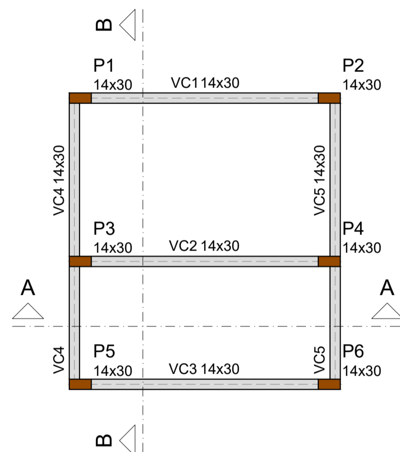
FORMA COBERTURA (NÍVEL 270) ESC.: 1:50
