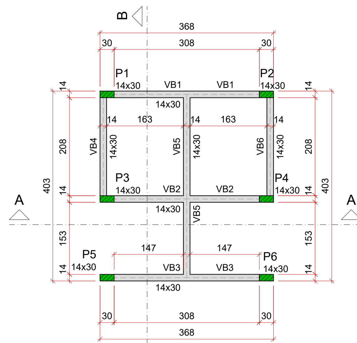
FORMA BALDRAME (NÍVEL 0) ESC.: 1:50
