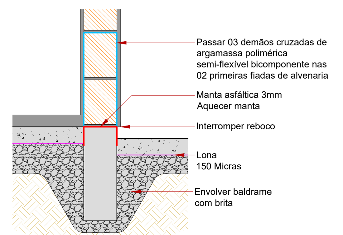
IMPERMEABILIZAÇÃO ESC.: 1:10
