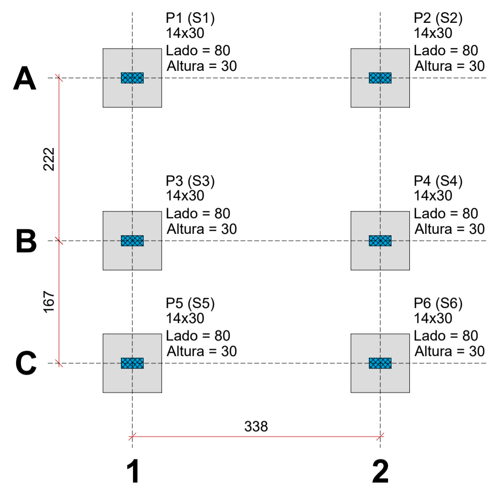
PLANTA DE LOCAÇÃO ESC.: 1:50
