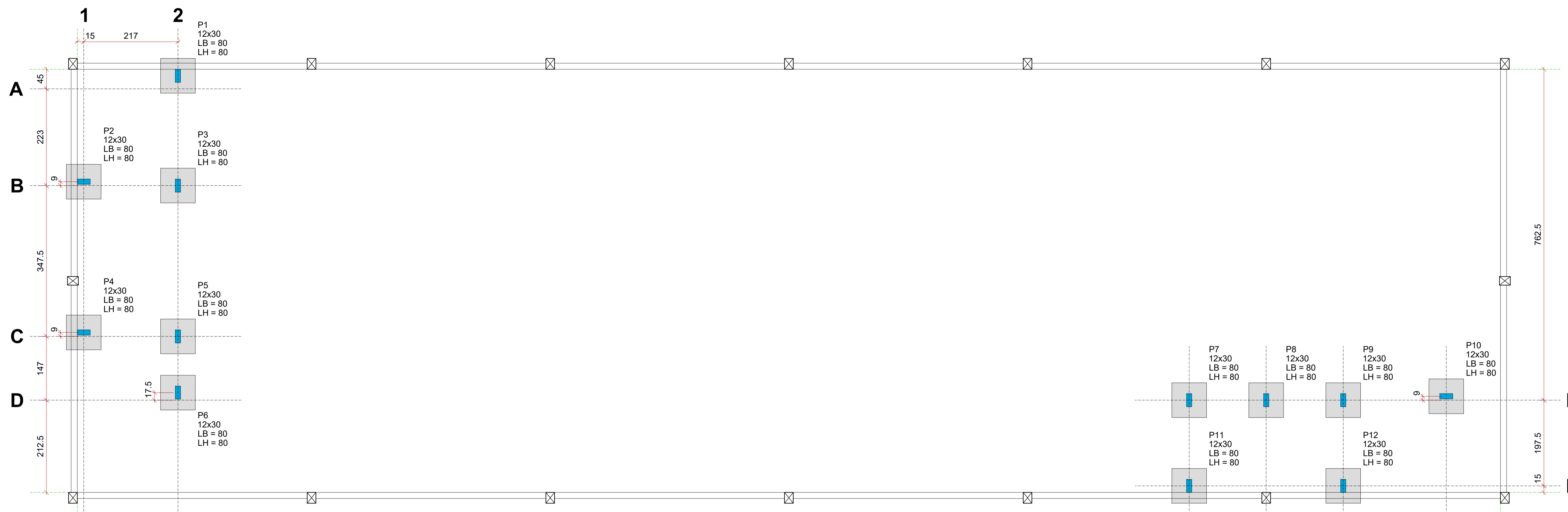
PLANTA DE LOCAÇÃO - ÁREA DE SERVIÇO E BANHEIROS ESC.: 1:50
