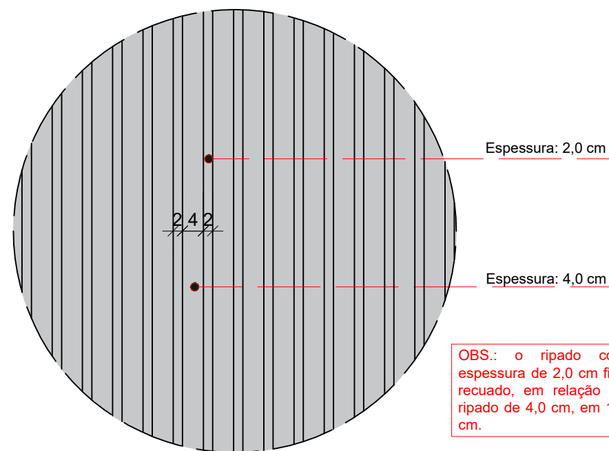
DETALHE 02 - RIPADO
