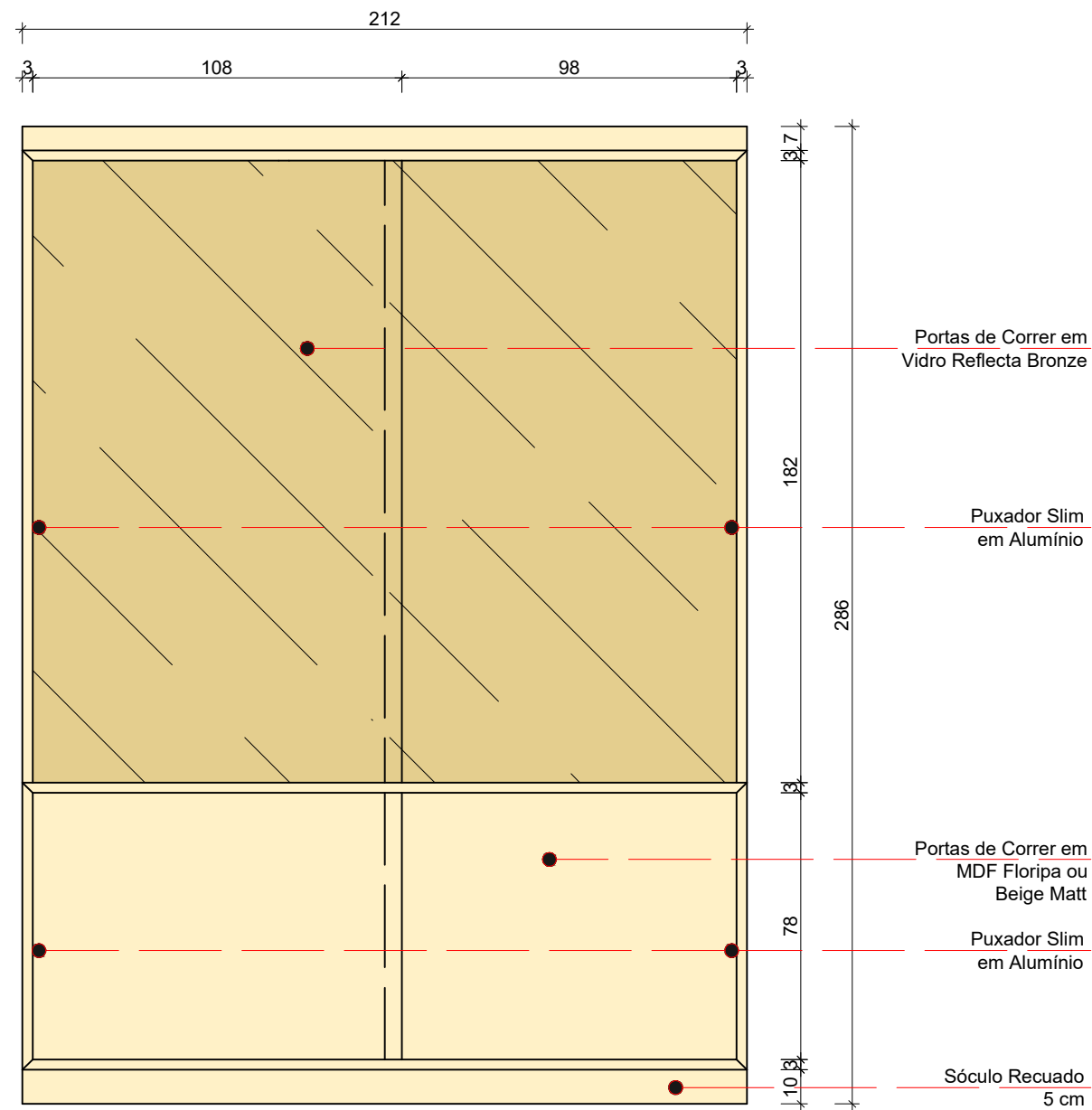
VISTA FRONTAL SEM PORTAS ESC.: 1/20
