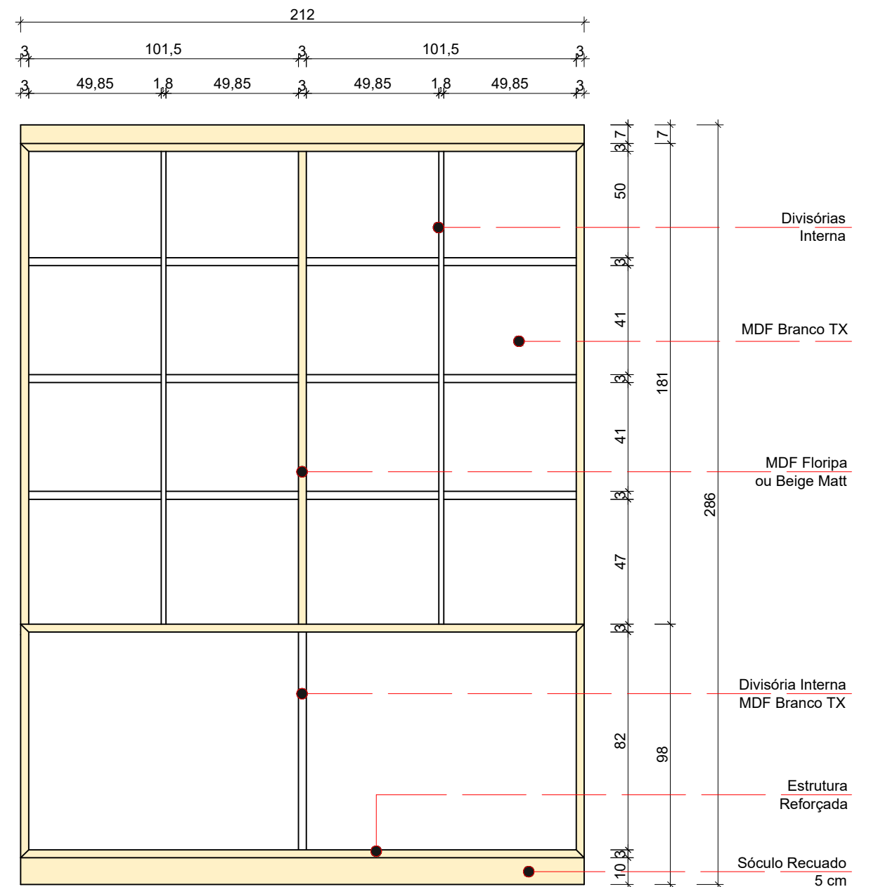
VISTA FRONTAL COM PORTAS ESC.: 1/20
